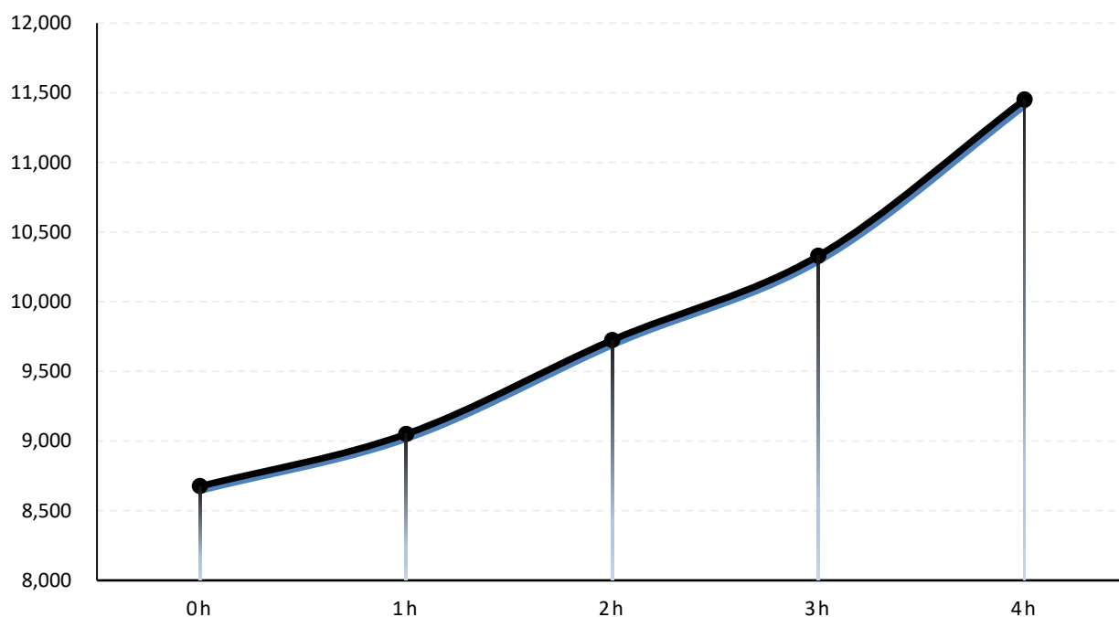
图二 FC3310T热稳定性曲线 (80 °C)
