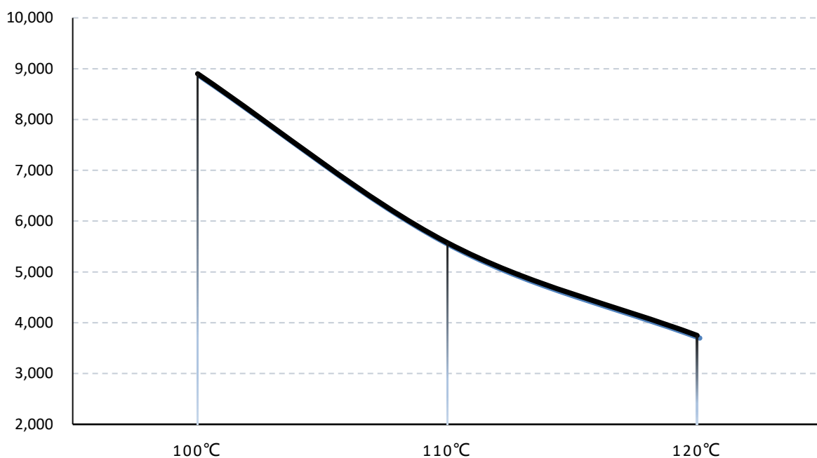
图1 FG3291 温度-粘度曲线
