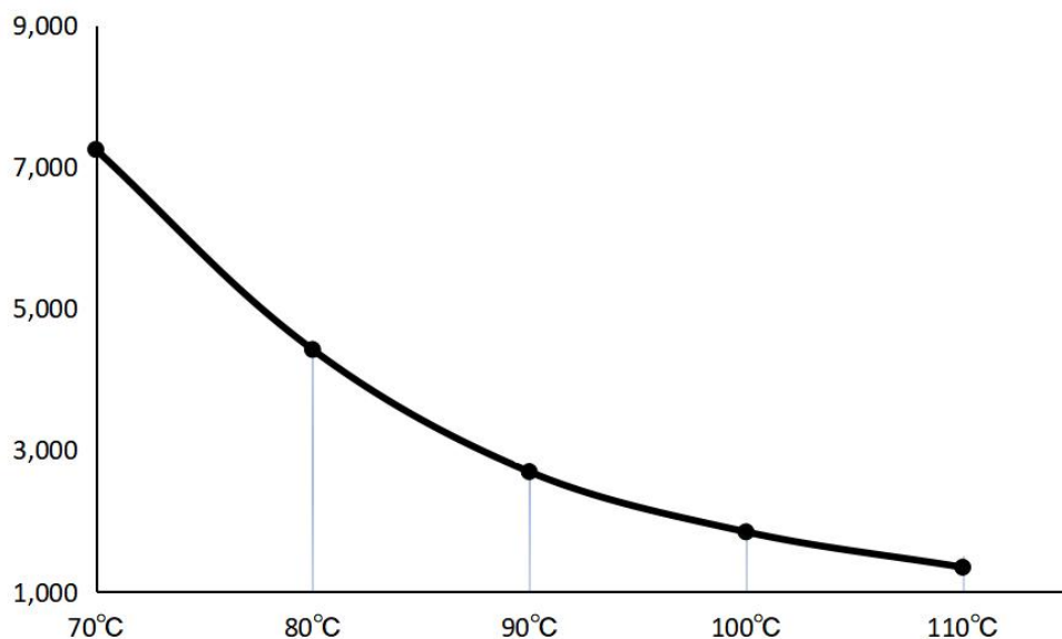
图一 FG3276-2 温度-粘度曲线
