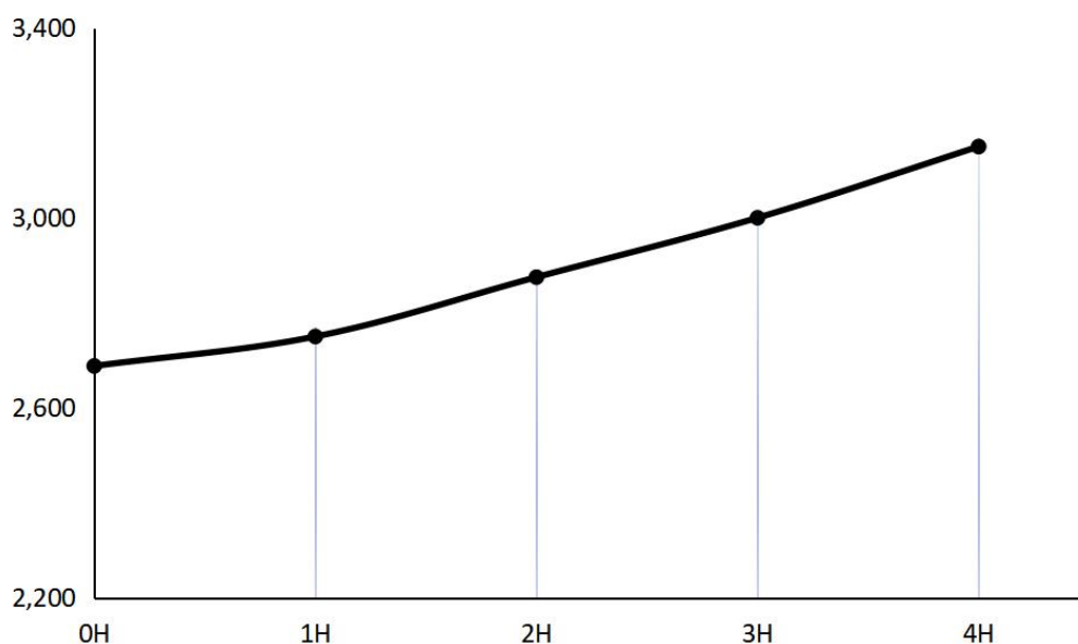
图二 FG3276-2热稳定性曲线 (90 °C)
