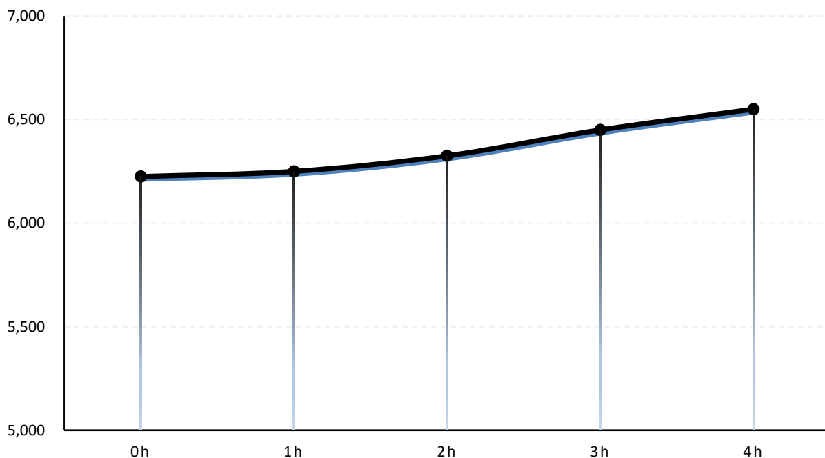
图二 FG3206热稳定性曲线 (80 °C)
