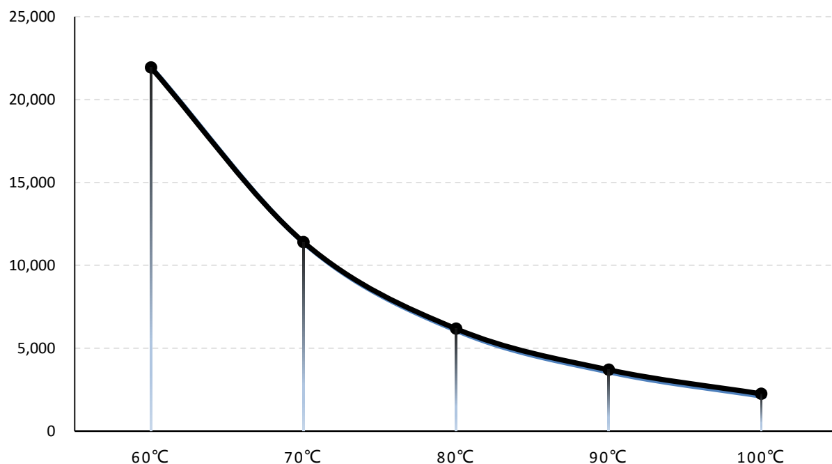
图一 FG3206 温度-粘度曲线
