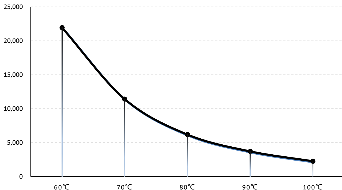
图一 FG3208 温度-粘度曲线
