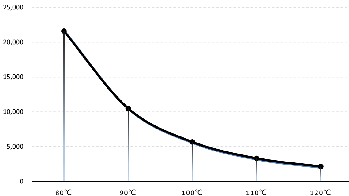
图一 FN3108GA 温度-粘度曲线
